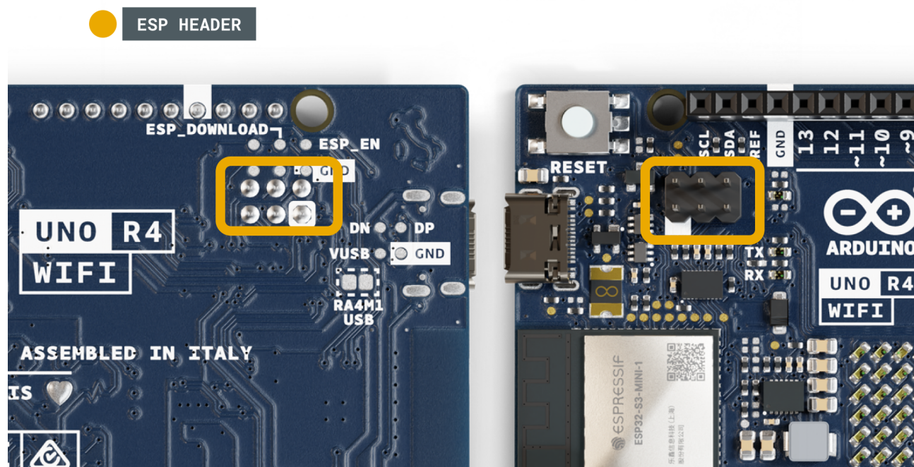
ESP针脚
