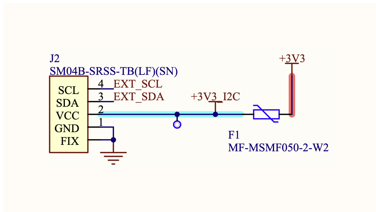
I2C连接器。
